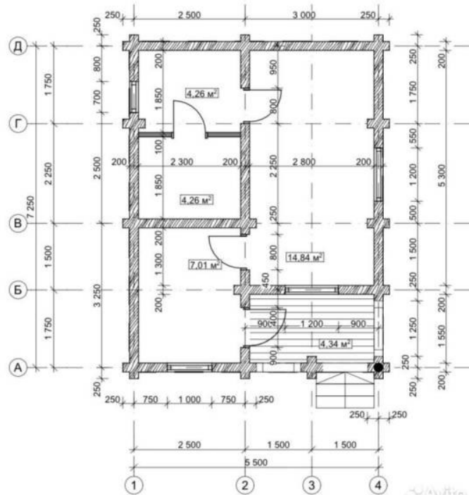
План 1 этажа
